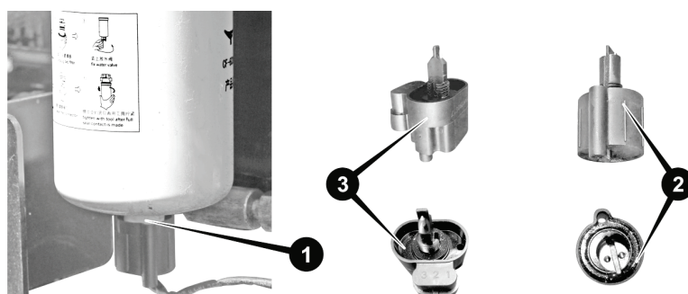
Рисунок 3.8. Відмінності фільтра грубої очистки палива
