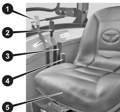
Рисунок 4.6. Важелі управління гідророзподільником
