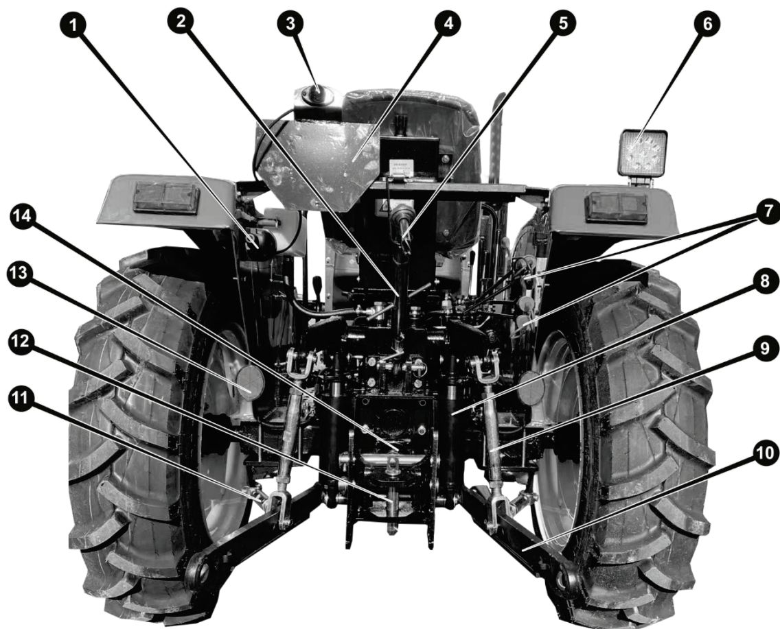
Рисунок 3.5. Триточкова гідронавісна система і вал відбору потужності
