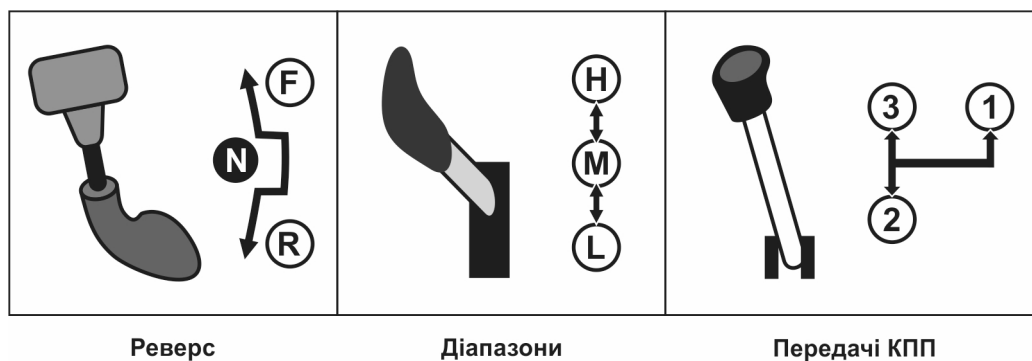
Рисунок 4.1. Перемикання передач
