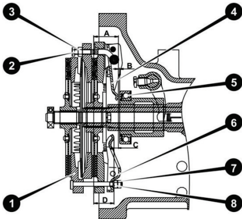
Рисунок 6.2. Муфта зчеплення дводискова
