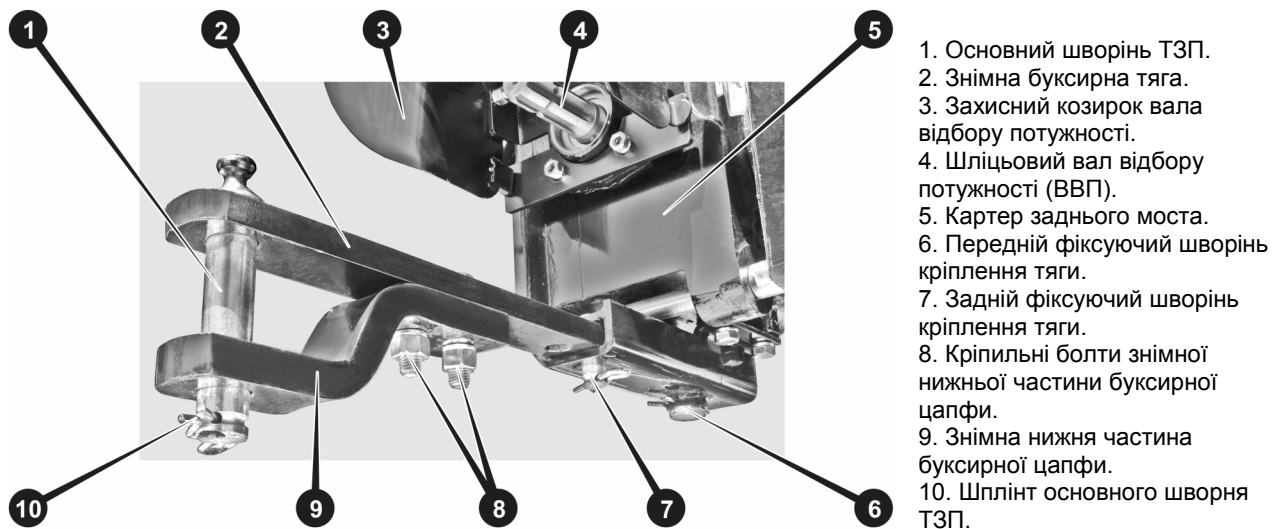
Рисунок 5.2. Тягово-зчіпний пристрій
