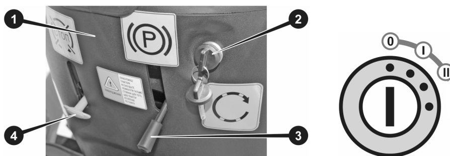
Рисунок 3.8. Центральний вимикач («замок запалювання»)
