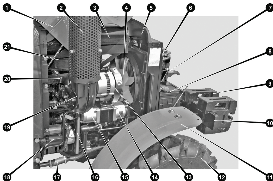
Рисунок 3.4. Двигун CF3B35T, вид справа
