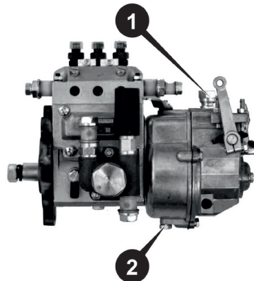
Рисунок 6.1. – Заливний (1) та зливний (2) отвори мастила ПНВТ
